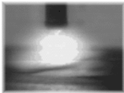
Pulsad svetsning
