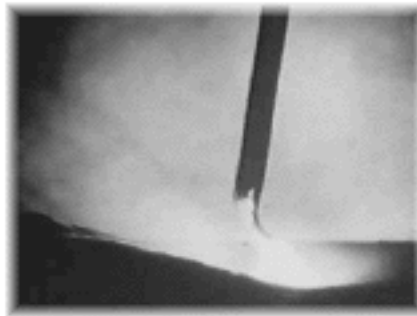
Roterande ljusbåge
